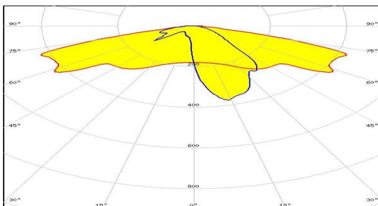
Диаграмма направленности
