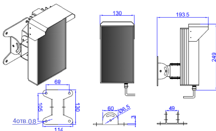
Пржектор с креплением В1
