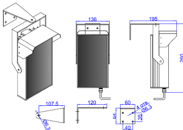
Пржектор с креплением В2
