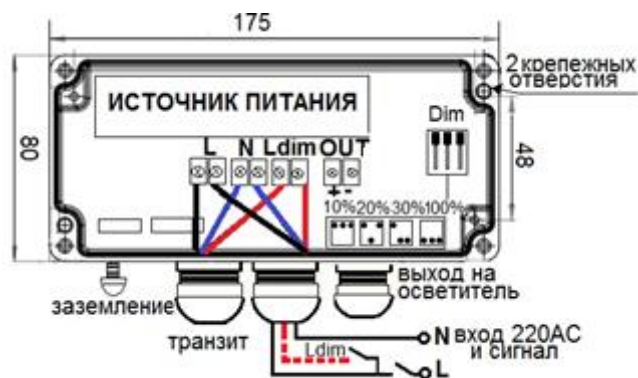
Блок питания и управления
